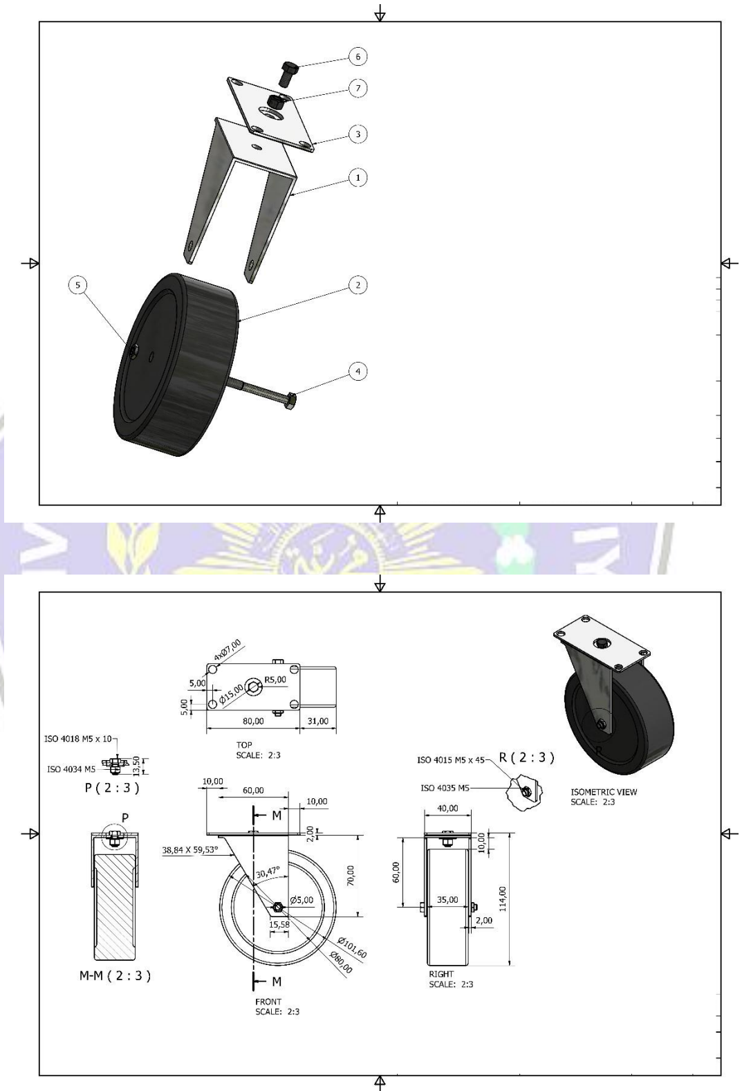
Gambar Komponen Roda Nilon 4 Inch Beserta Dimensi
