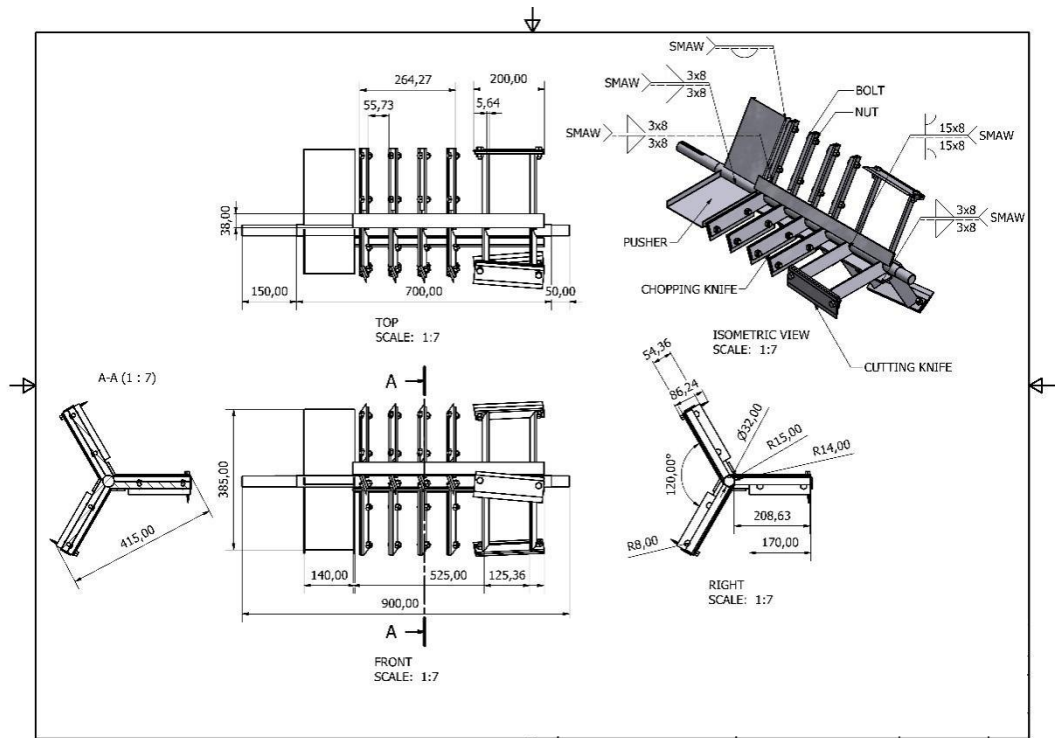
Gambar Komponen Pisau Beserta Dimensi
