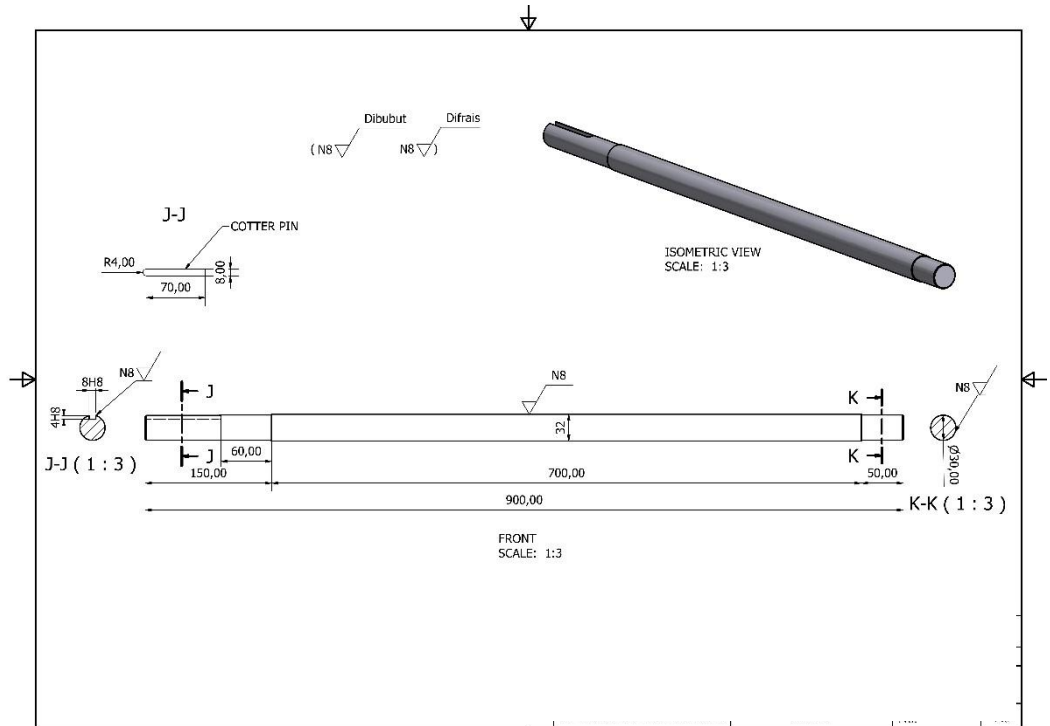
Gambar Komponen Poros dan Bantalan Beserta Dimensi
