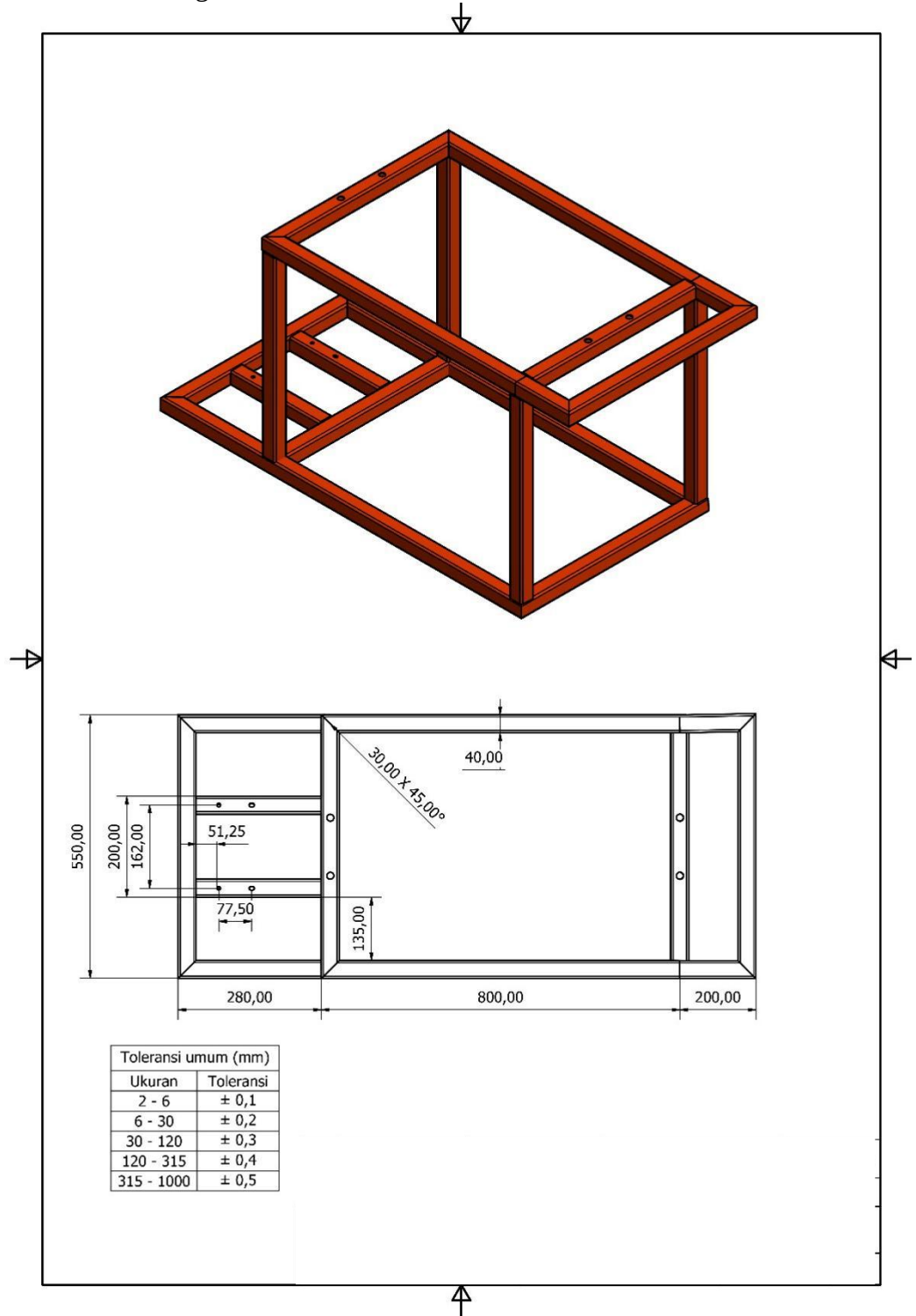
Gambar Rangka Beserta Dimensi
