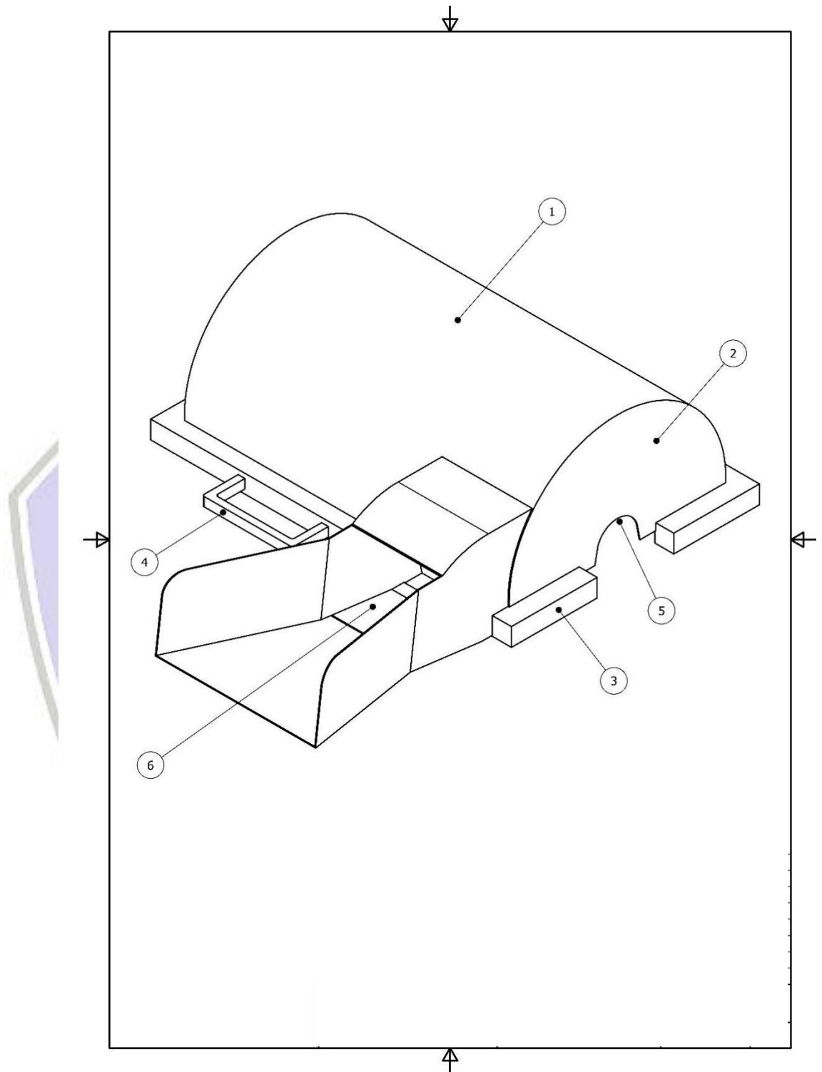
Gambar Komponen Tabung Atas dan Bawah Beserta Dimensi
