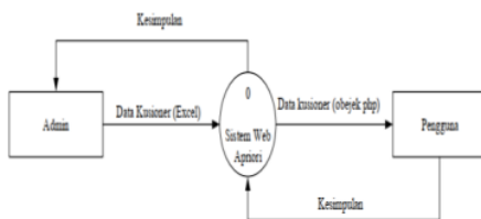
Gambar 6. Diagram Konteks
