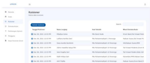
Gambar 5 Tambah Kusioner
