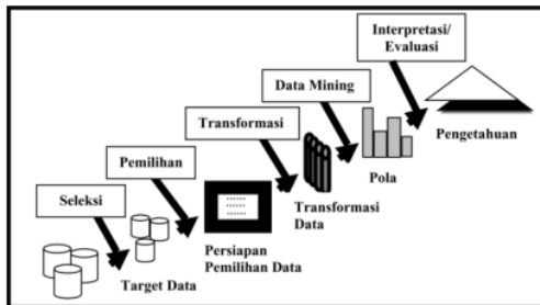
Gambar 1.Proses Tahapan KDD ((Syahril et al., 2020)
