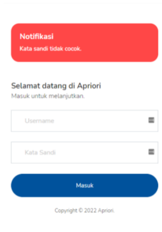
Gambar 3 Halaman Login
