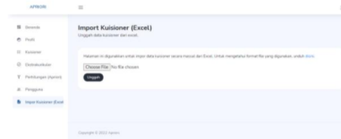
Gambar 6 Import Kusioner
