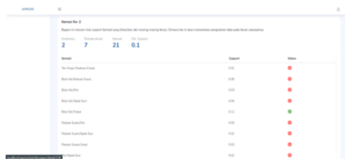
Gambar 10. Iterasi ke-2
