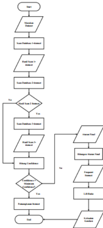
Gambar 5 Flowchart Apriori
