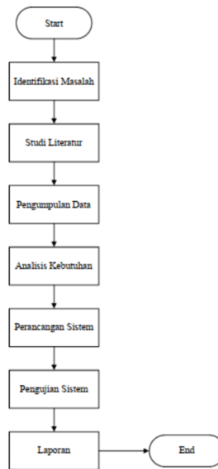
Gambar 3. Tahapan Penelitian
