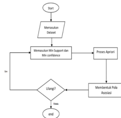
Gambar 1. Flowchart Perancangan
