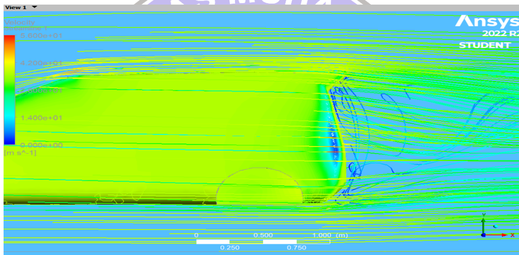
Desain Spoiler B Ketika Simulasi
