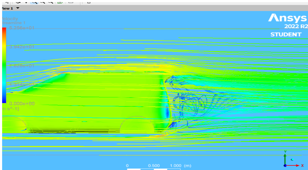
Desain Spoiler A Ketika Simulsi
