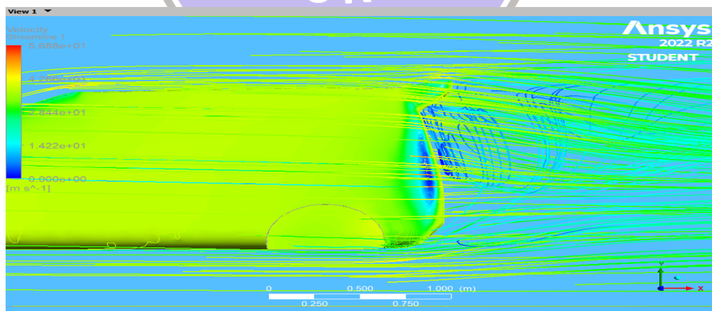
Desain Spoiler C Ketika Simulasi
