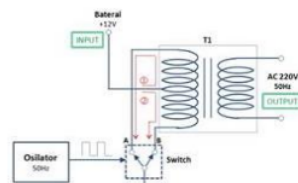
Gambar 6. Inverter fasa tunggal
