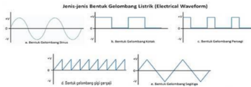
Gambar 5. Berbagai bentuk gelombang yang dapat dihasilkan inverter .
