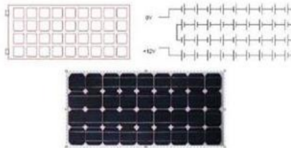
Gambar 2. Modul surya terdiri dari 28-36 sel surya
