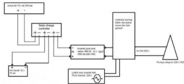
Gambar 8. Skema sistem listrik Hibrid untuk pompa air
