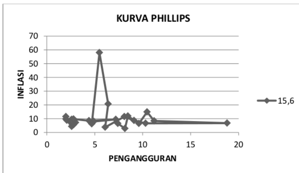
Gambar 2. Pengujian Kurva Philips untuk Indonesia (tahun 1981-2010)
