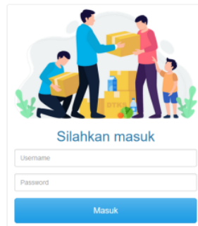
Gambar 3: Halaman Login
