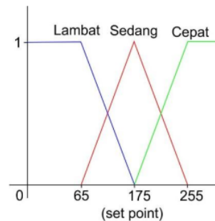
Gambar 3. Output keanggotaan kipas
