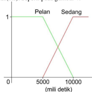
Gambar 4. Output Waktu Pompa
