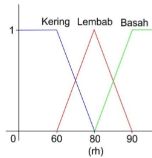
Gambar 2. Keanggotaan kelembapan udara
