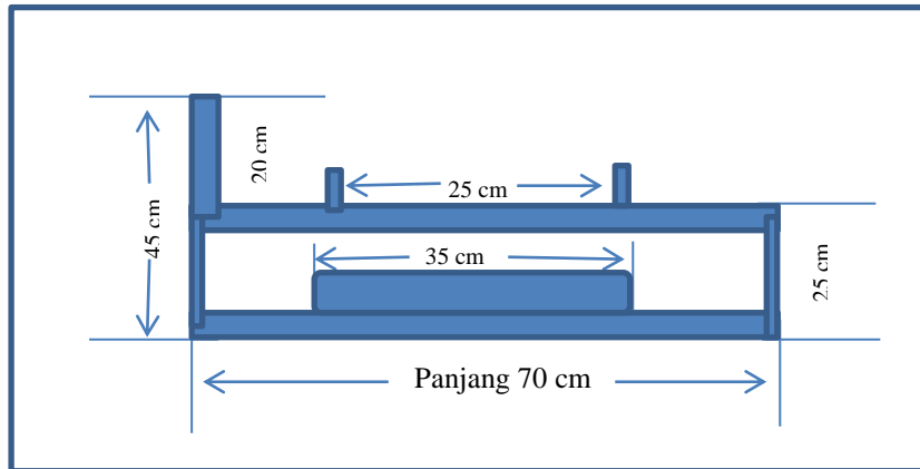
Gambar landasan konstruksi Nampak dari samping
