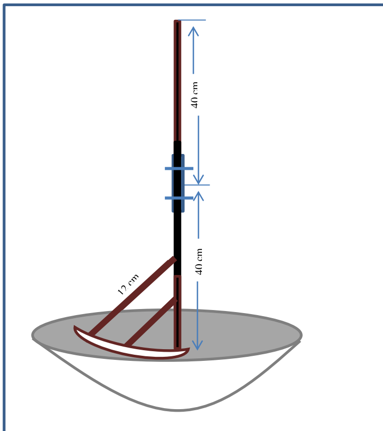
Gambar lengan pengaduk konstruksi Nampak dari samping
