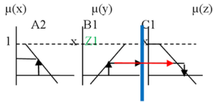
Gambar 2 Inferensi fuzzy menggunakan metode Tsukamoto (Jang, 1997)
