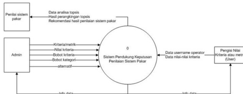
Gambar 3. Diagram Konteks Sistem
