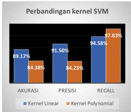
Gambar 13 Hasil Perbandingan Kernel SVM
