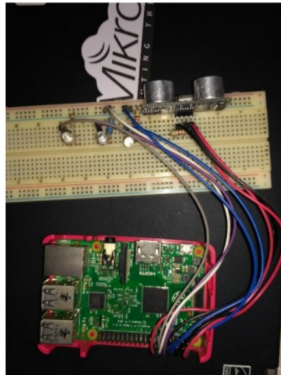
Gambar 1. Sensor ultrasonik yang terhubung pada raspberry pi
