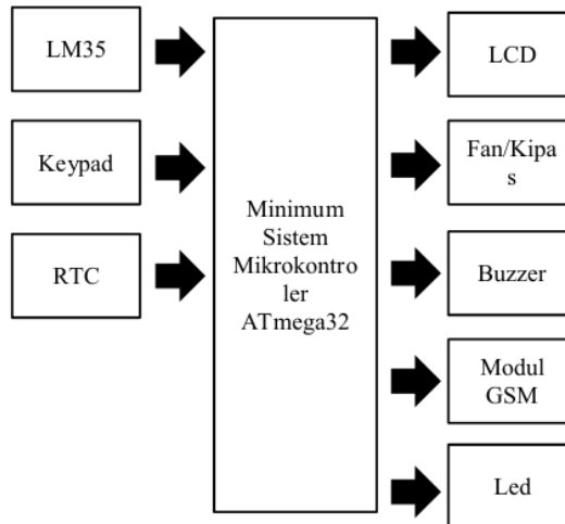
Gambar 1. Blok Diagram Perangkat Keras
