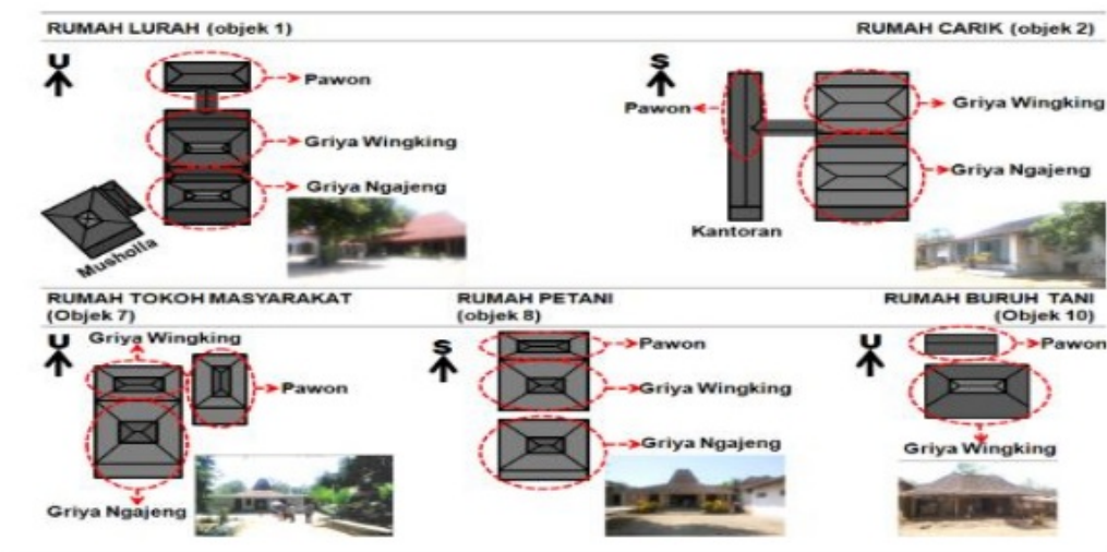
Gambar 4 Organisasi Ruang pada Rumah Jawa Panaragan Sumber: diolah dari (Yunita Nurmayant, 2017)
