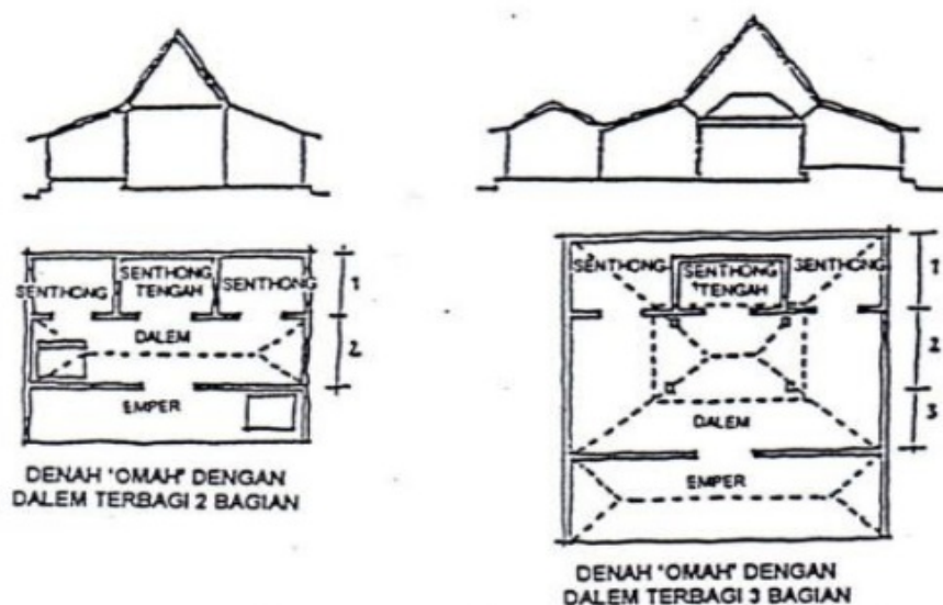
Gambar 1 Unit - unit dalam rumah Jawa Sumber diolah dari: (Waheni, 2017)
