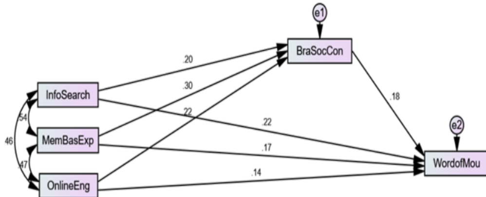
Figure 5: SEM
