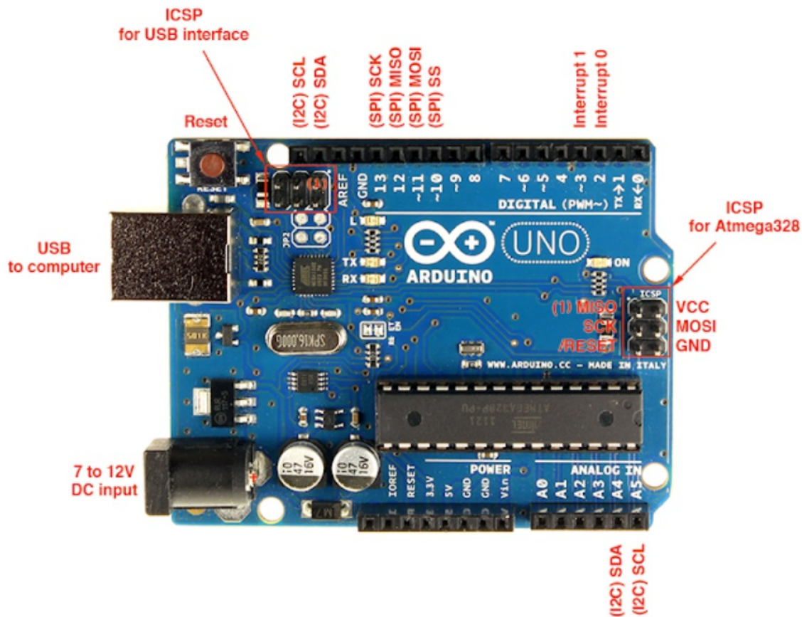
Figure 2. Arduino uno 3
