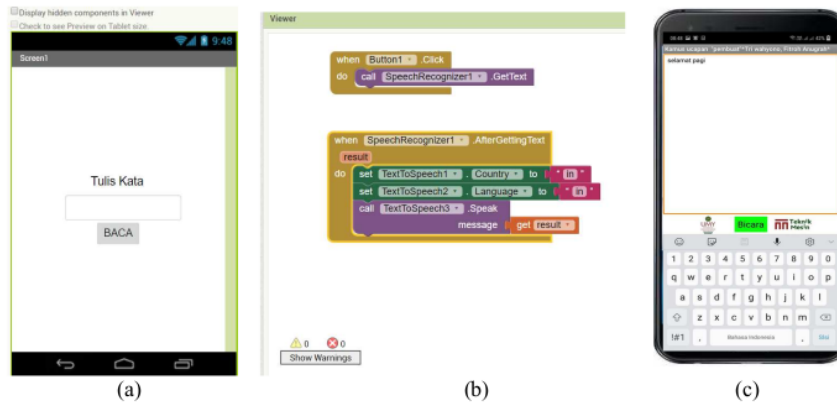
Gambar 3. Alur perancangan aplikasi: (a) Tampilan desain dari project Kamus Bersuara bahasa Indonesia, (b) Block Code dari aplikasi Kamus Bersuara bahasa Indonesia, (c) Tampilan Aplikasi Kamus Suara Bahasa Indonesia
