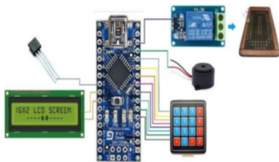
Gambar 2 Rangkaian sistem keseluruhan Keterangan:
