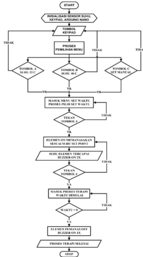
Gambar 2 Flowchart sistem keseluruhan
