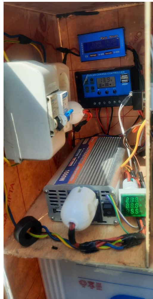
Komponen PLTS
