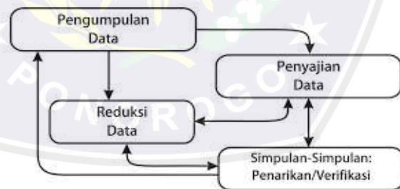
Gambar 2. Tahap-tahap Analisis Kualitatif
